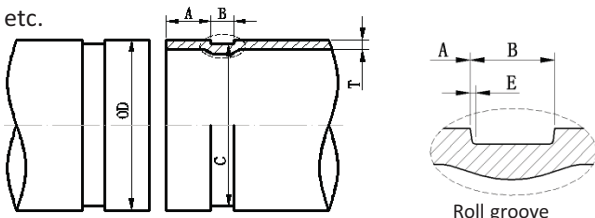
Roll groove
